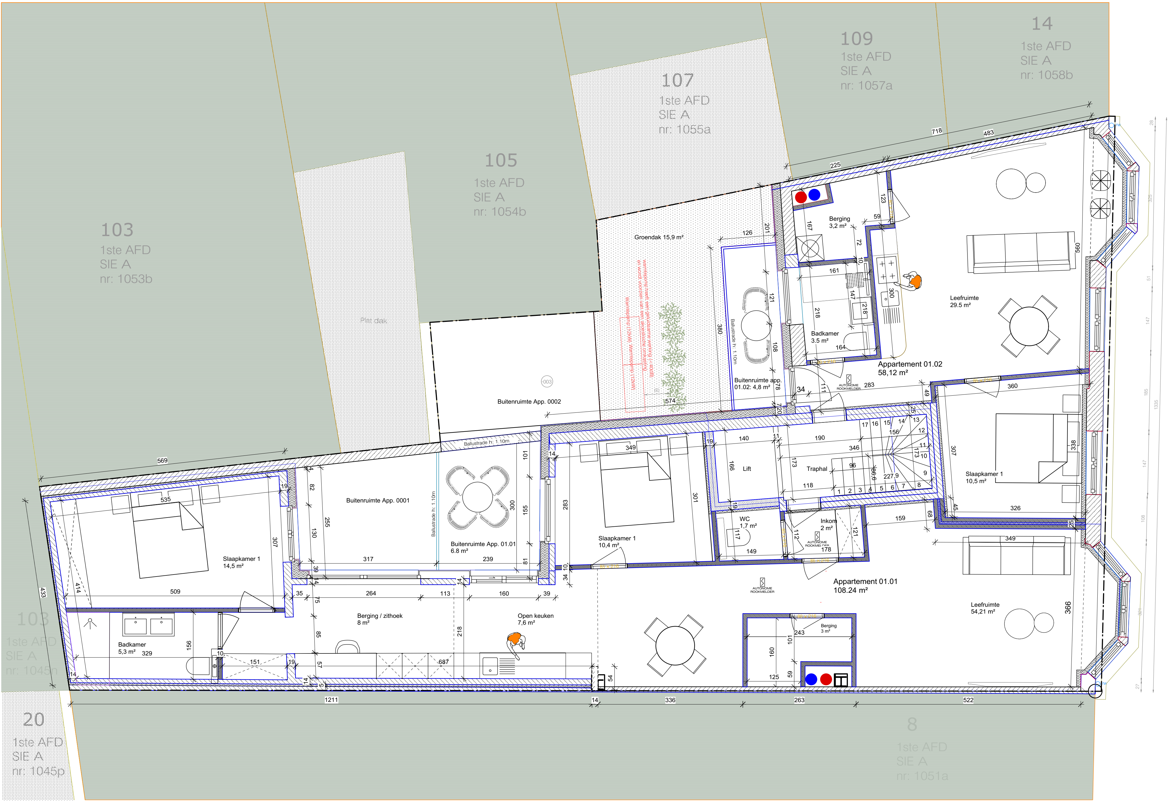
Grondplan Verdiep 1
